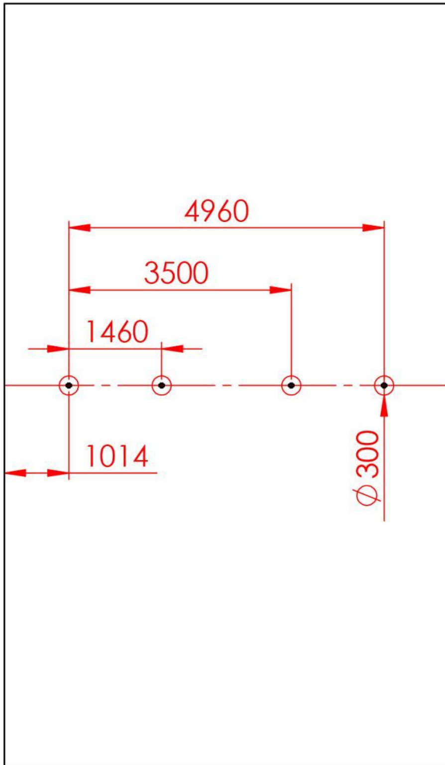
1. Plaatsing gaten Soccer44 (maten in mm)
