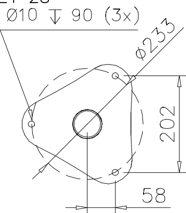
DET 31
