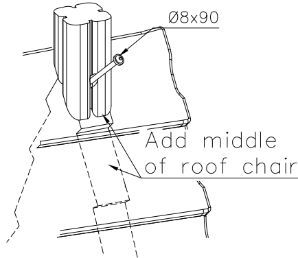
DET 8
